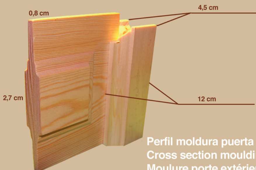
Perfil moldura armario Cross section moulding cupboard Moulure porte d'armoire
